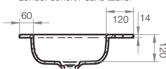
zonder schort / sans tablier
