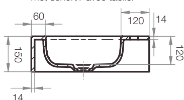
section A-A met schort / avec tablier
