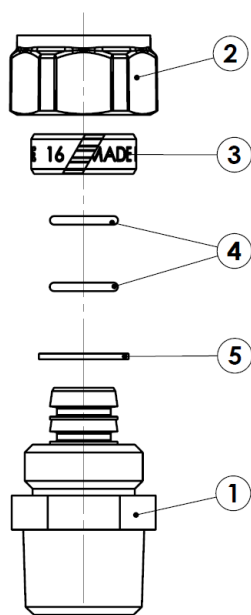
Fig. 1 – Onderdelen van de klemkoppeling
