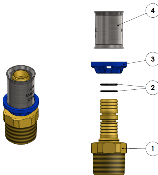
Fig. 2 – Onderdelen van de perskoppeling
